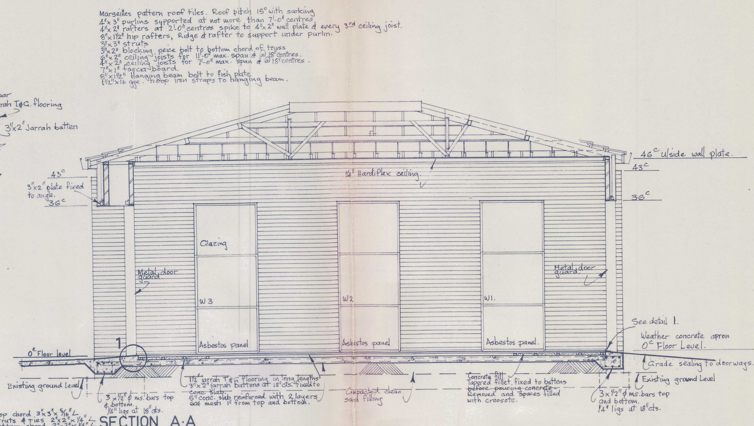
SECTION A-A
